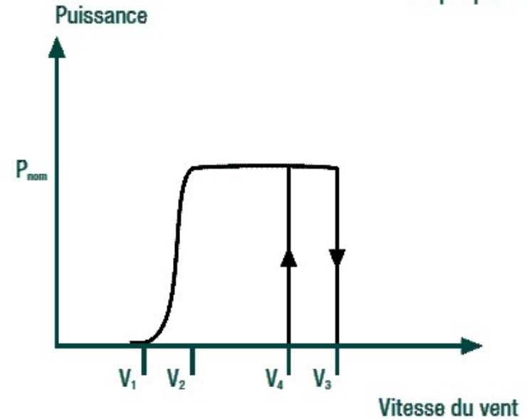
Courbe de puissance sans mode tempête ENERCON
