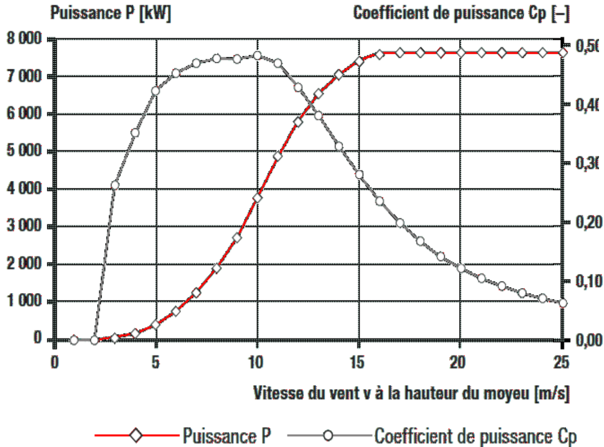
Courbe de puissance sans mode tempête ENERCON
