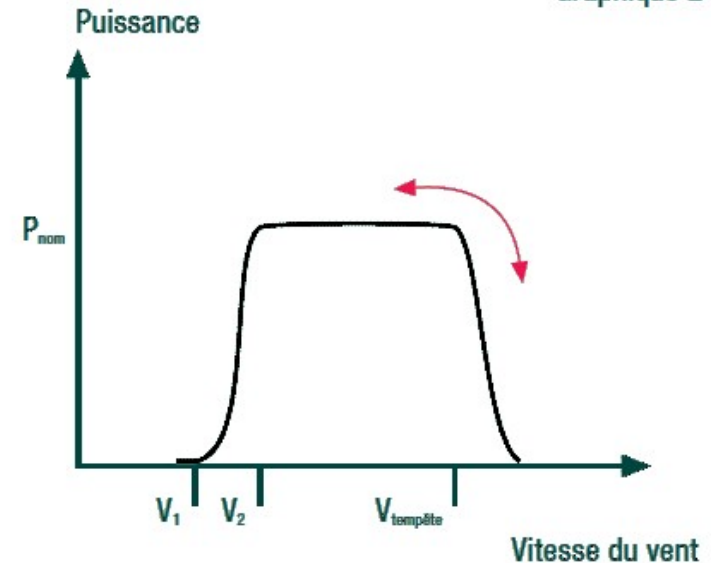
Courbe de puissance avec mode tempête ENERCON
