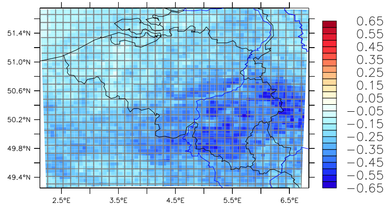
MAR-NORhisto (1976-2005)
