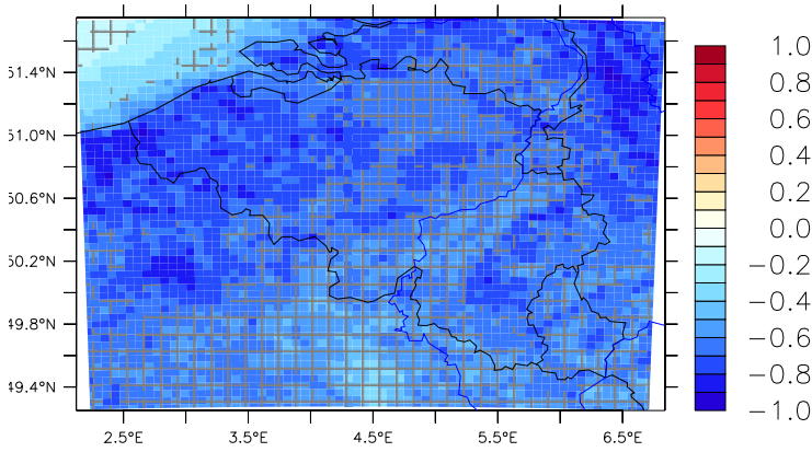
MAR-MIRhisto (1976-2005)
