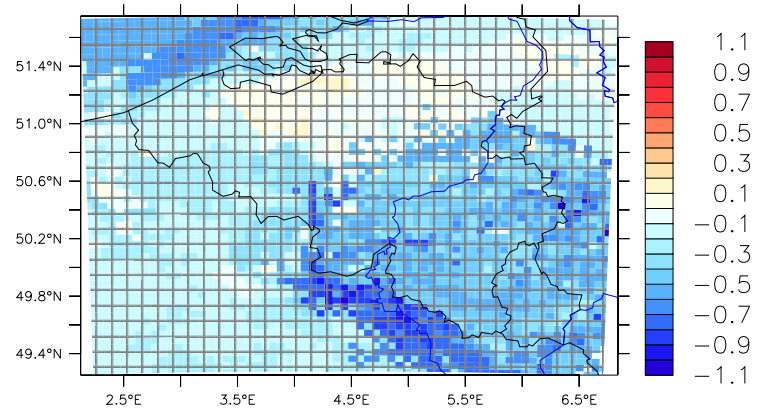
MAR-NORhisto (1976-2005)
